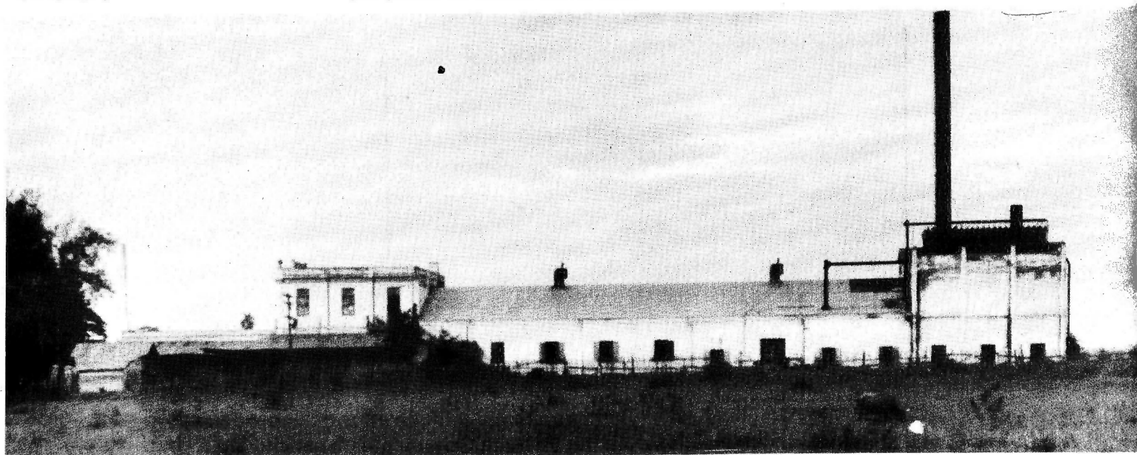
PLANTA DE HIELO "LA NACIONAL".—Situada en la carretera de Guanabacoa, con una superficie de 102,459.64 metros cuadrados, con capacidad para producir 125 toneladas cada 24 horas.
