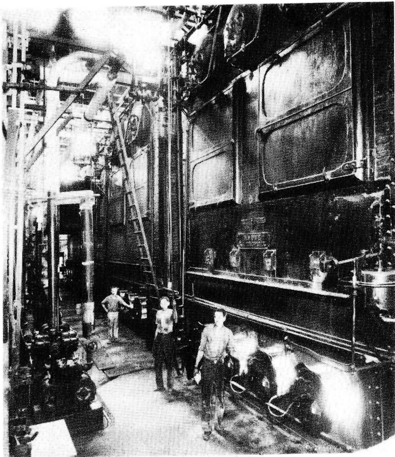
Baterías de calderas equipadas para combustible de petróleo, compuestas por cuatro calderas "Babcock and Wilcox", de 600 C. F. cada una, o sean 2,400 C. F. en total.
