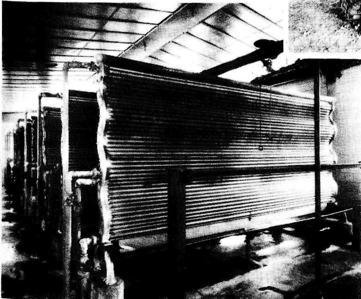
Enfriadores de mosto, todos de cobre. En la mitad superior son enfriados los mostos que corren por su exterior con agua por dentro, fresca a la temperatura ambiente, y también por dentro de su mitad inferior circula salmuera a la temperatura por debajo de congelación, y de aquí pasan los mostos, ya enfriados, a la Bodega de Fermentación.
