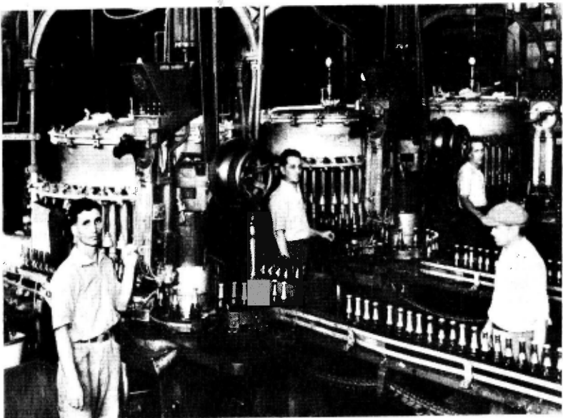
Máquinas de llenar y tapar, con capacidad para 50,000 botellas cada máquina en 8 horas. Cada colonia tiene 2 máquinas de cada una de éstas.
