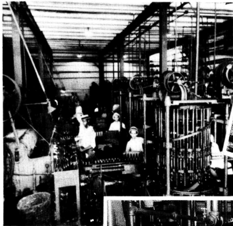
SALIDA DE LAS BOTELLAS DE LOS SUMERGIDORES.—A la izquierda se ven éstas pasando por los cepillos de lavado exterior, y a la derecha las botellas pasan por la máquina de lavar de cepillos interiores y enjuague.
