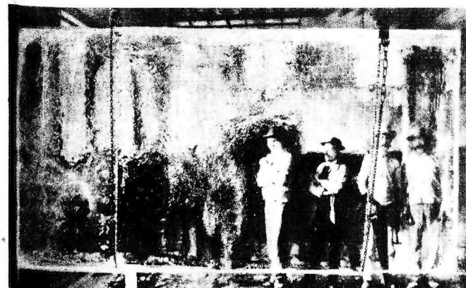
Fotografía a través de un bloque de hielo de 5 toneladas. Planta de 40 toneladas en funcionamiento en el año 1914.
