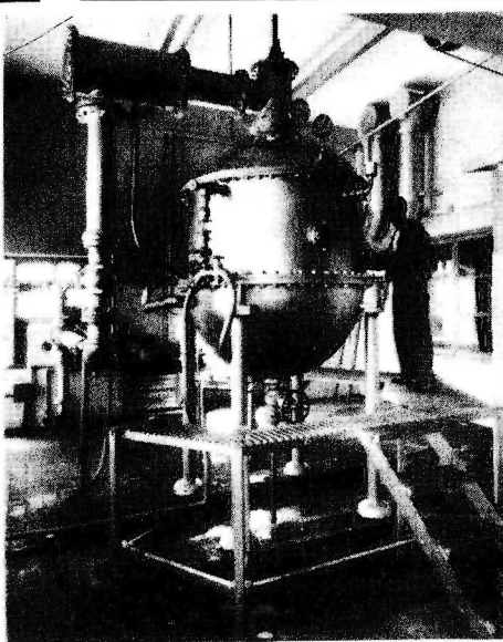
Tacho al vacío, para la preparación de los extractos vitamínicos que contienen las vitaminas A, B y D, que están dosificadas en nuestra "Maltina Tivoli Vitaminada"
