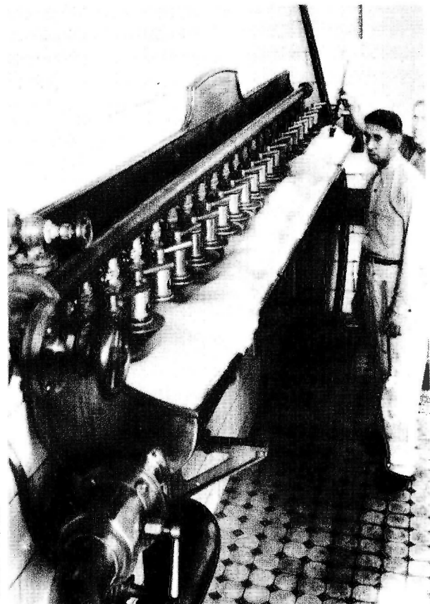
Bateria de boquillas de los Coladores de Mosto. Primeras manifestaciones de espuma de los mostos. Obsérvense la limpieza de los mismos por el bruñido que ostentan los metales.
